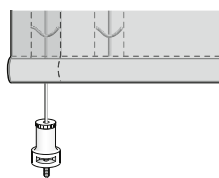
Pendelsicherung Mit Schnur Ø 1,4 mm, weiß, Standard 50 mm von außen.
