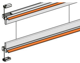
04-2050 S. 14 - 17 AREO mit Griffleiste ↔ 20 cm - 150 cm ↓ 220 cm
